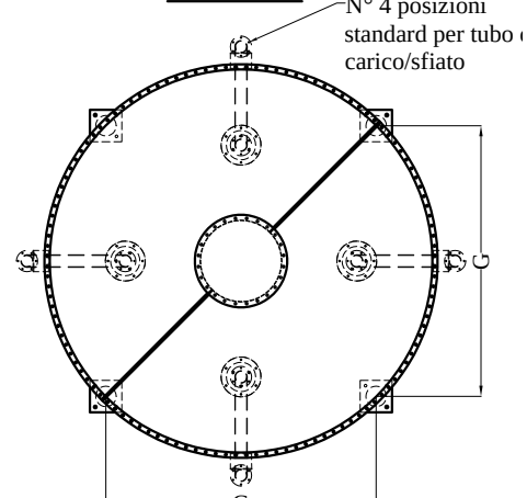
PLANTA SILOS
