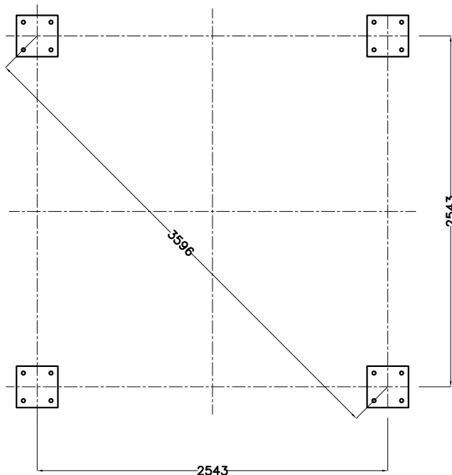
PIANTA DI FONDAZIONE
