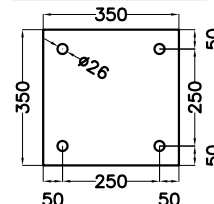
PIASTRA DI FONDAZIONE TIPO "B"
