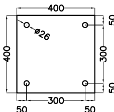
PIASTRA DI FONDAZIONE TIPO "C"
