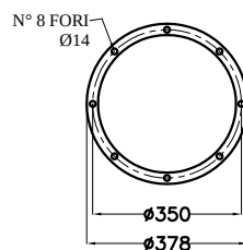
FLANGIA FINALE TUBO DI CARICO
