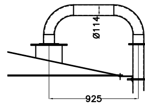
CURVA TUBO DI SFIATO
