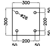
PIASTRA DI FONDAZIONE TIPO "A"
