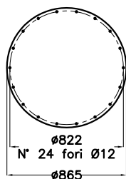
PREDISPOSIZIONE PER FLUIDIFICAZIONE STANDARD
