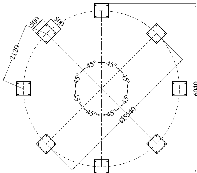
PIANTA DI FONDAZIONE
