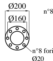
FLANGIA FINALE TUBO DI CARICO
