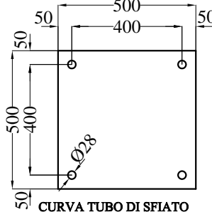
CURVA TUBO DI SFIATO
