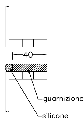
GUARNIZIONE TIPICA
