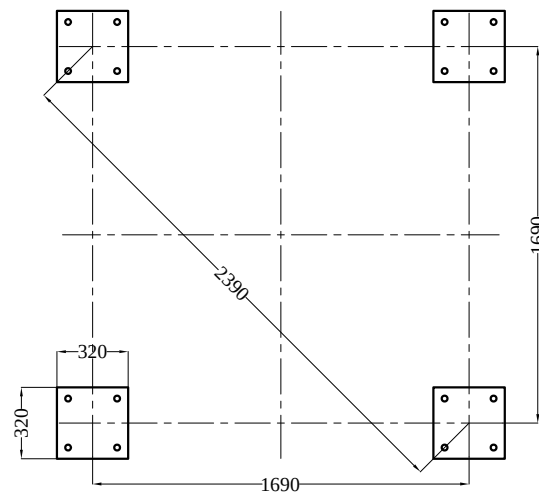
PIANTA DI FONDAZIONE
