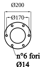
FLANGIA INTERMEDIA TUBI DI CARICO
