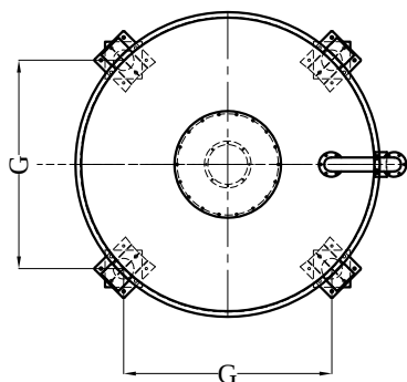
PIANTA SILOS
