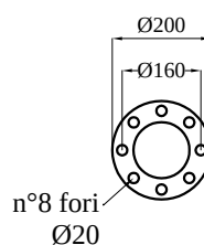
FLANGIA FINALE TUBO DI CARICO
