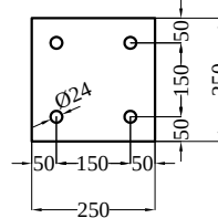
PIANTA SILOS
