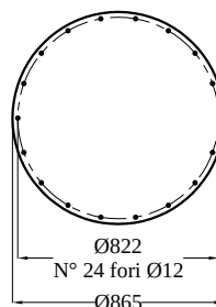
FORATURA SU TETTO SILOS
