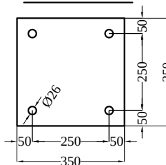
PIASTRA DI FONDAZIONE PER SILOS S=0
