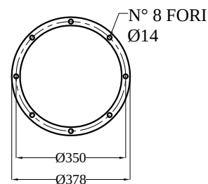
FLANGIA DI USCITA CONO SILOS
