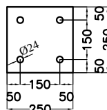
PIASTRA DI FONDAZIONE TIPO "A"
