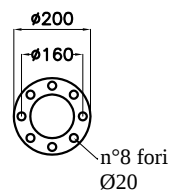
FLANGIA FINALE TUBO DI CARICO
