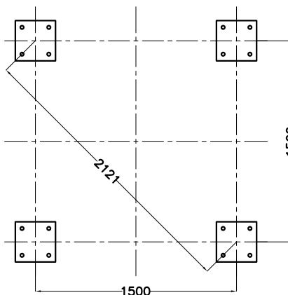
PIANTA DI FONDAZIONE
