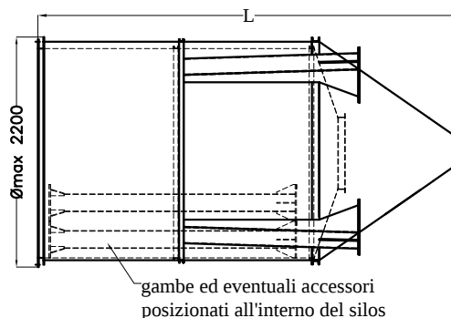
SCHEMA PER TRASPORTO
